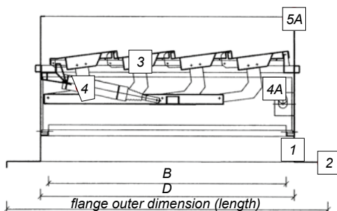
longitudinal section
